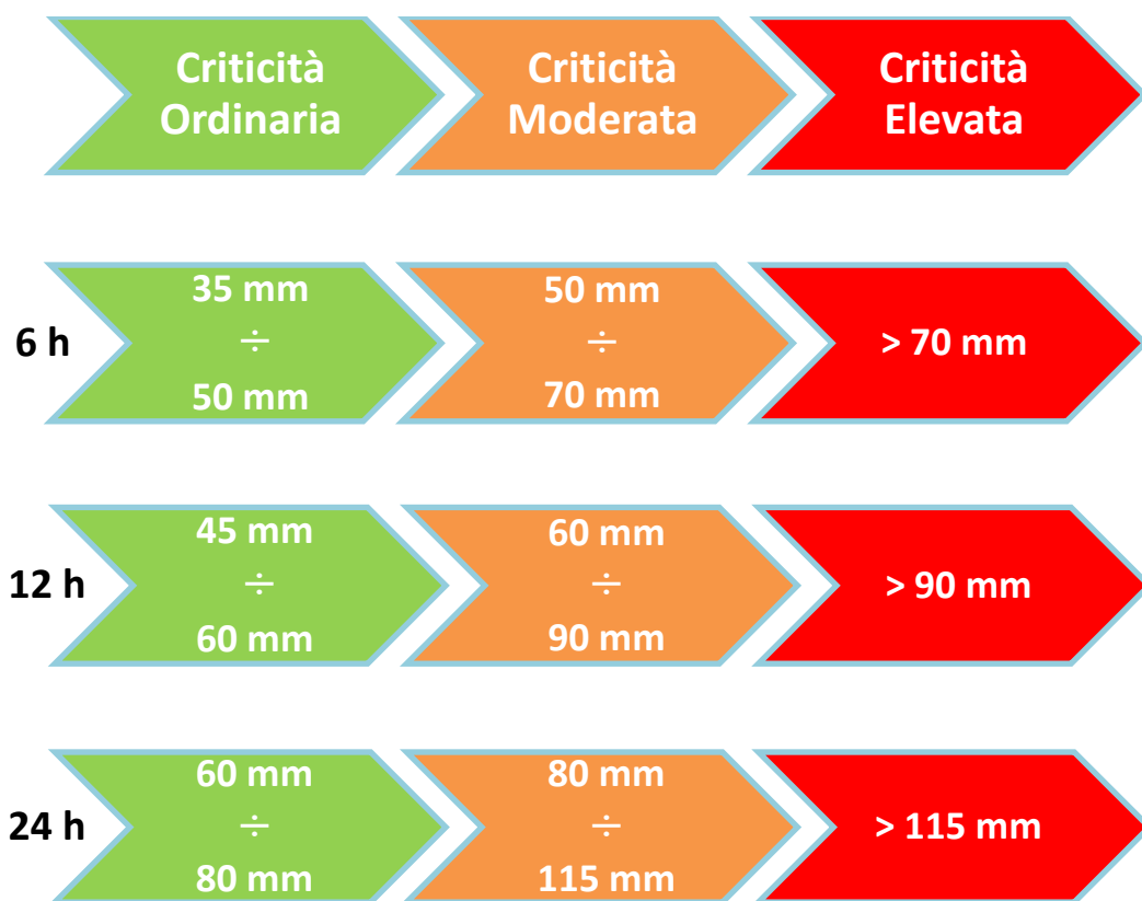
Figura 2 - Soglie per il rischio idrogeologico - idraulico suddivise per durata di precipitazione (6, 12 e 24 h) relative al Comune di Torre Boldone
